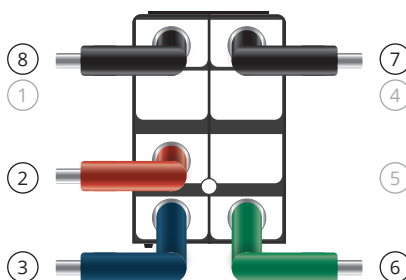
KABELBAUM (HINTEN)
