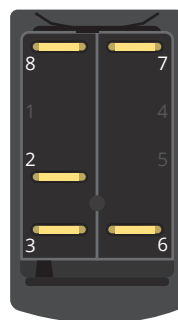
SCHALTER (HINTEN)
